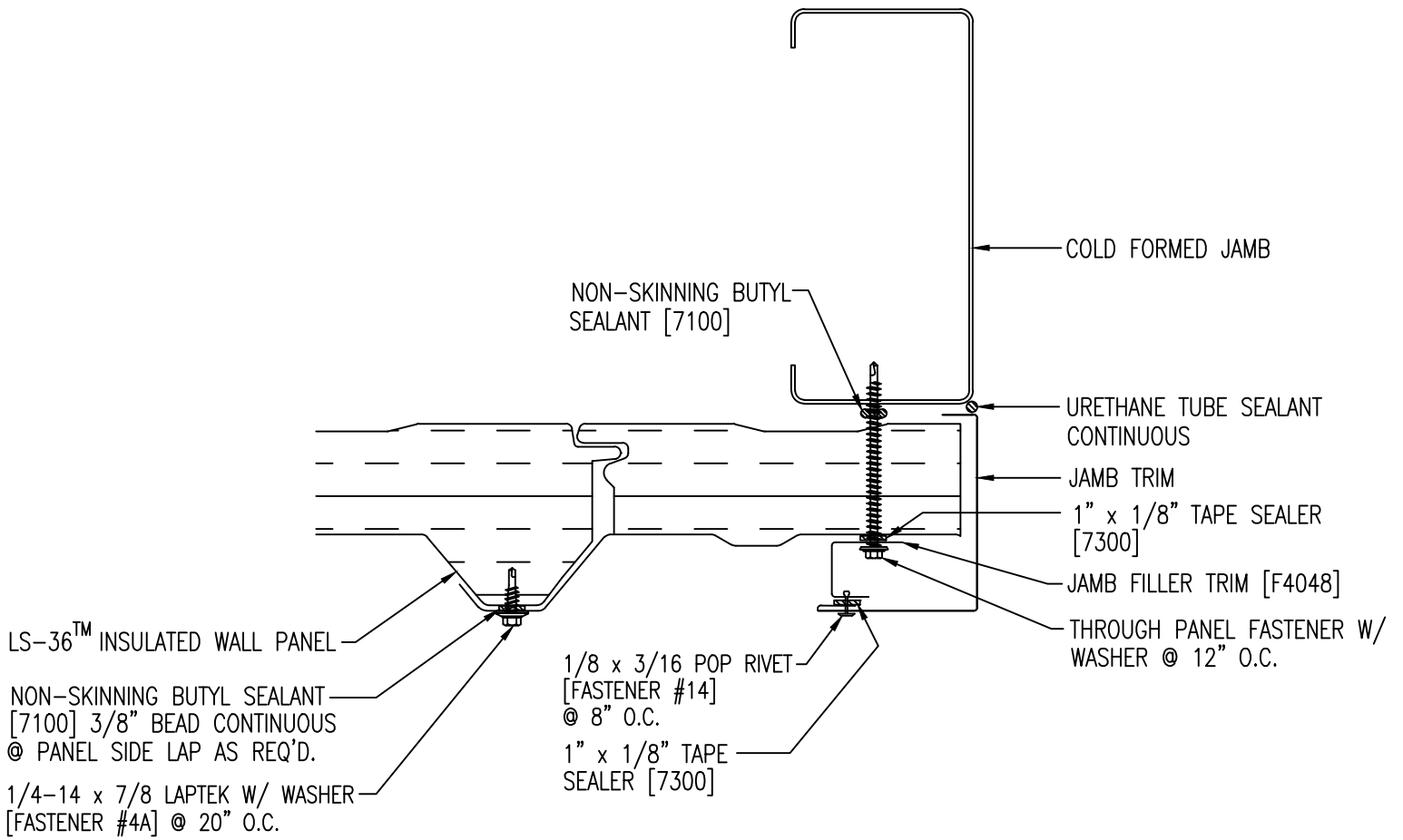
JAMB W/ JAMB FILLER TRIM
